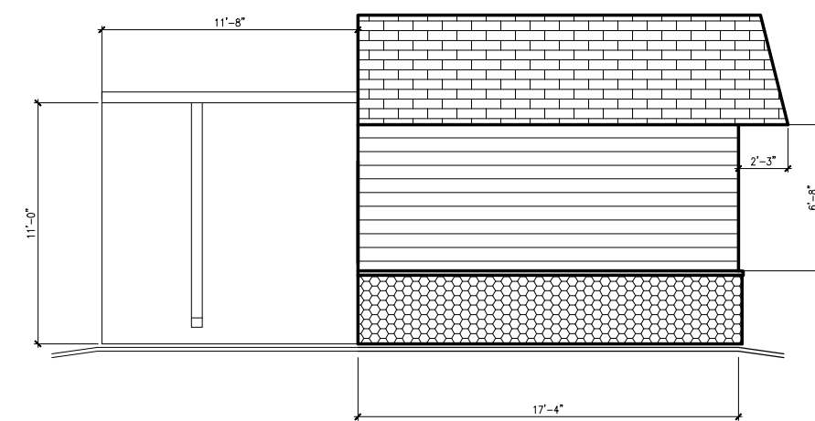
X 1 NEW Scale: 1/4" = 1'-0"
