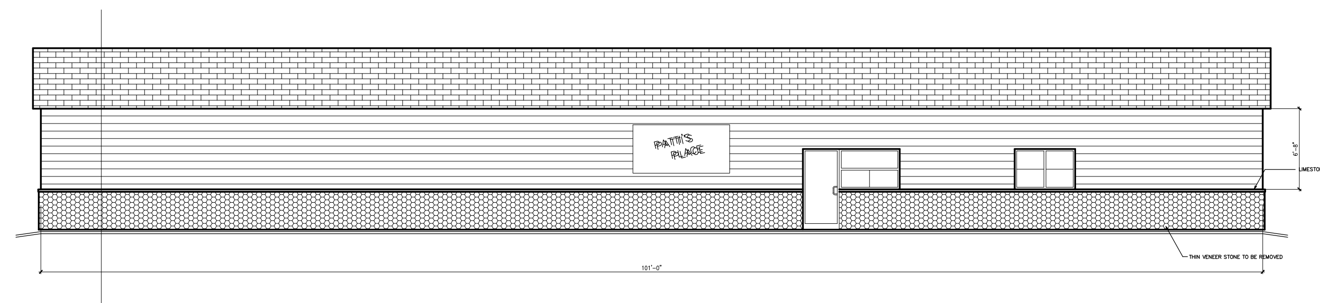
2 1 NEW Scale: 1/4" = 1'-0"
